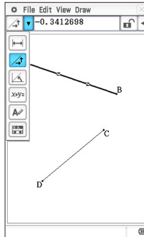
Gradient of AB
